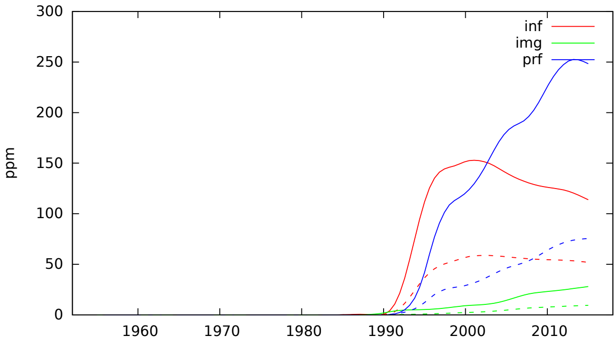
lemma_internet
