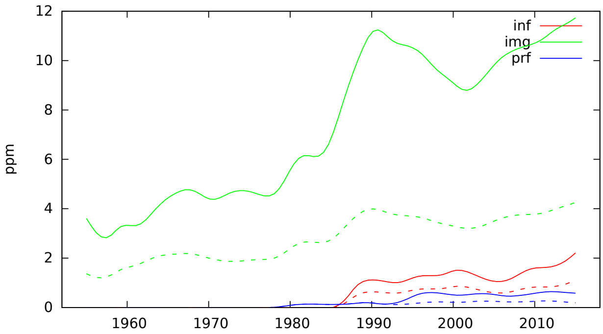
lemma_hovno
