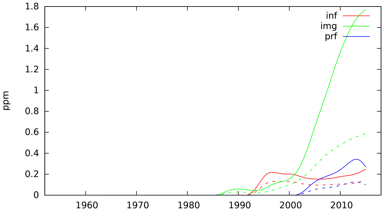
lemma_kokso
