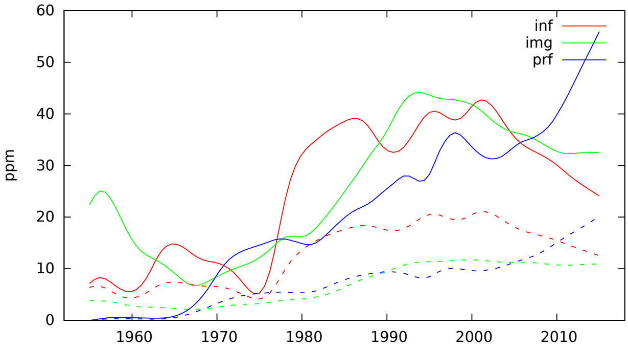
lemma_obrazovka
