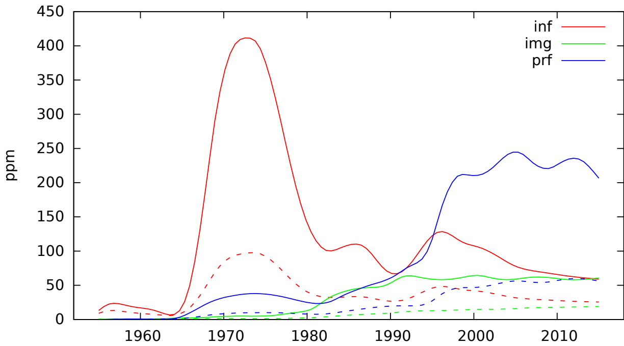
lemma_počítač
