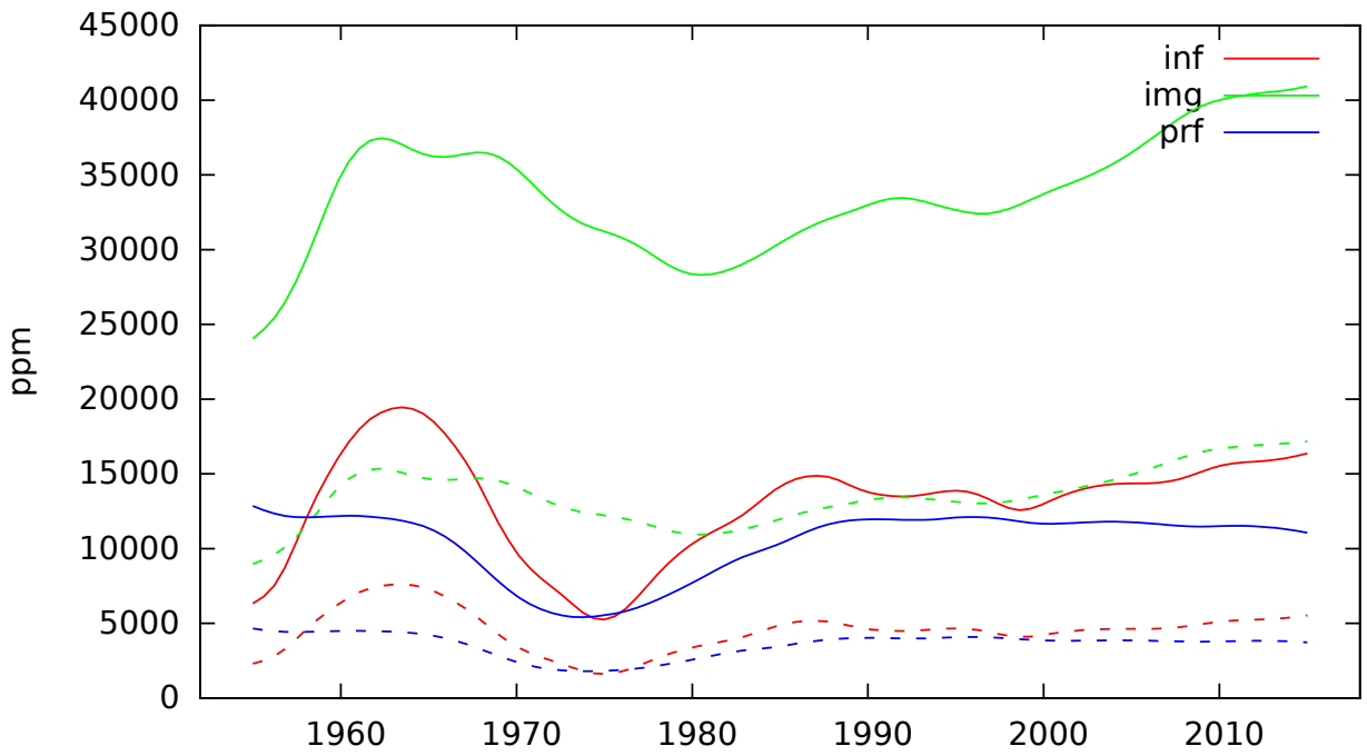
person_a
