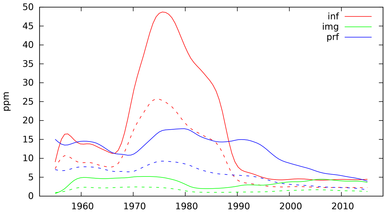
lemma_ruština
