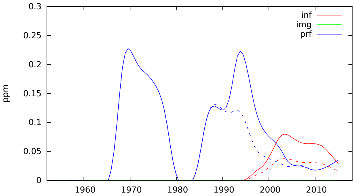
lemma_zamenhof
