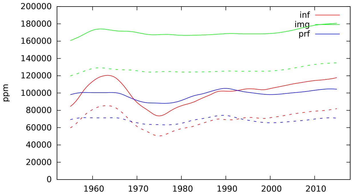
pos_V
