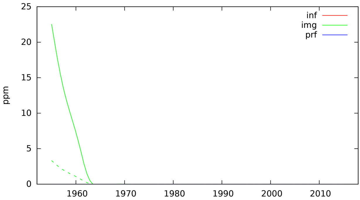
lemma_obraznica
